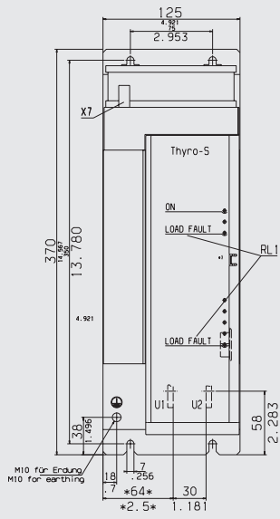
THYRO-S 1S (280H)
