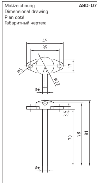
ASD-07 Anschlussnippel Connection nipple Embouts de raccordement Соединительный нипель
