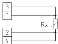
1x Vierleiterschaltung
