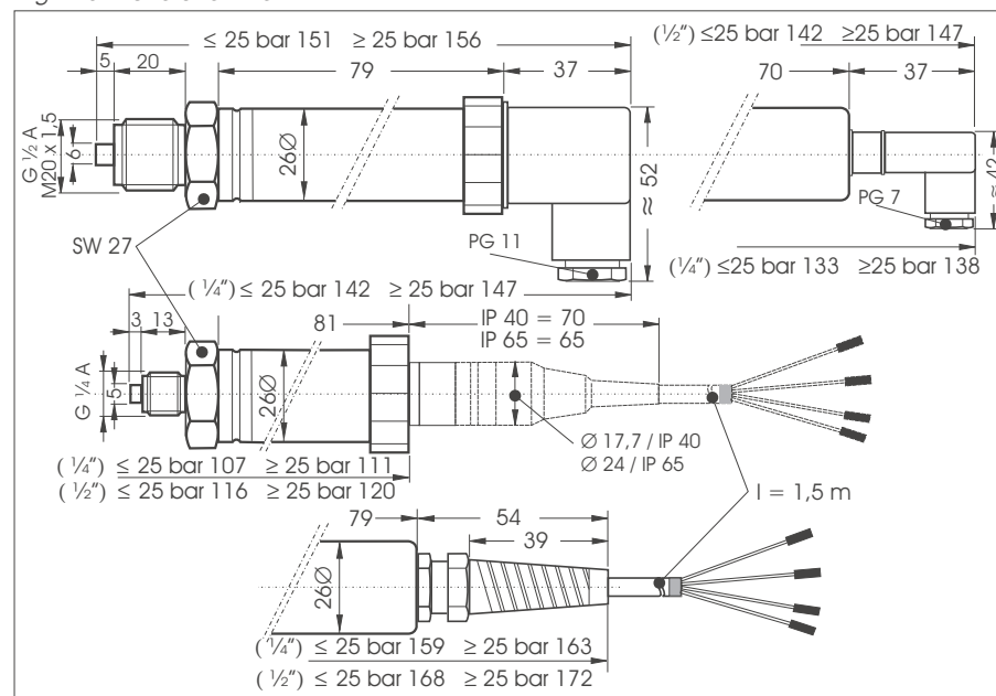
Fig. 2 dimensions P40
