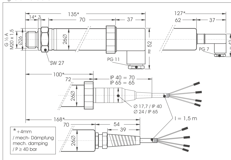
Fig. 3 dimensions P41
